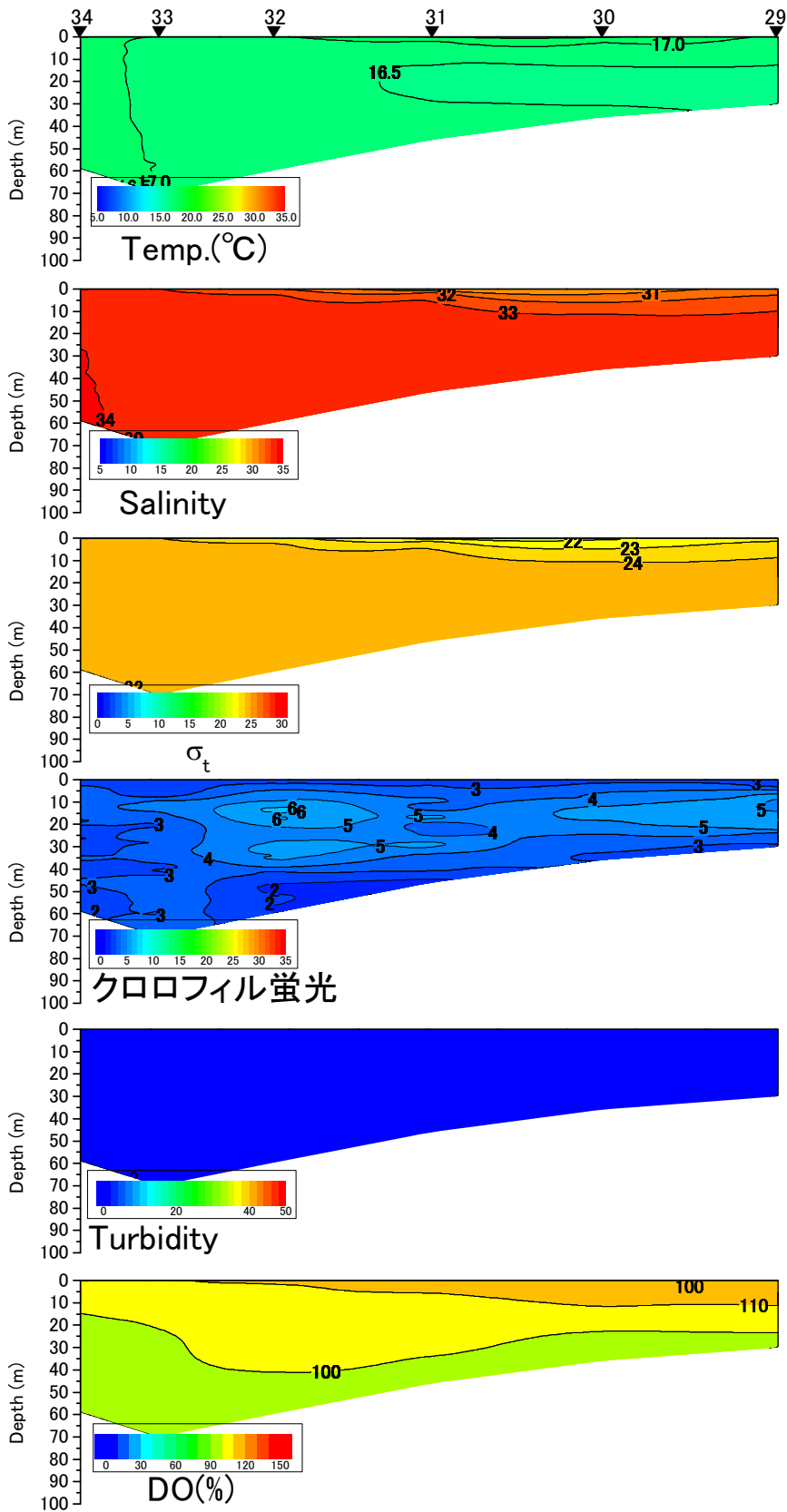
八代海西ラインの水温(°C)、塩分、密度( \sigma_t )、クロロフィル蛍光強度、濁度、溶存酸素飽和度(DO%)の鉛直面図(国土交通省の調査による) (2017年4月21日)
